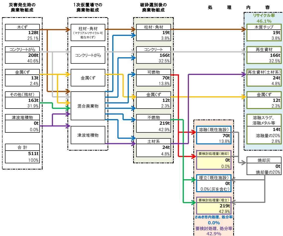
図 2-6-(3)-4 長尾断層の災害廃棄物処理フロー
