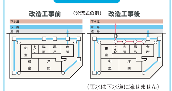
水洗化工事のモデル図
